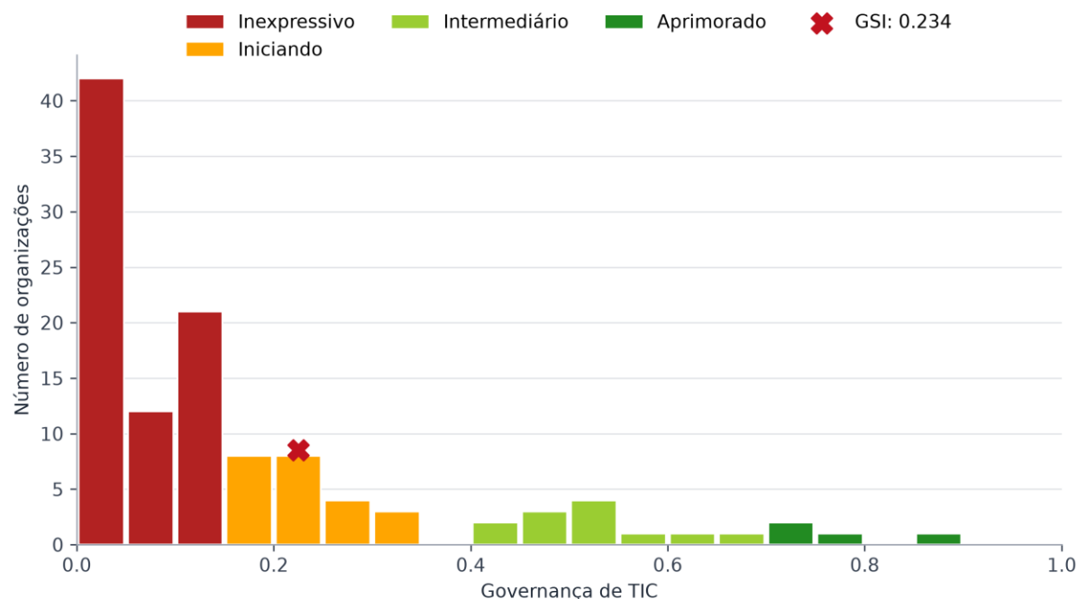
Figura 6 - Resultado do componente Governança de TIC da organização GSI
